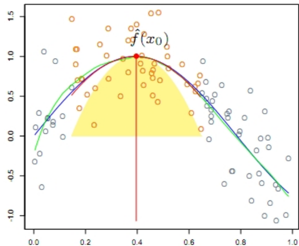
Квадратичная модель
