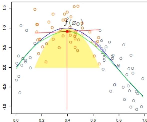
Линейная модель
